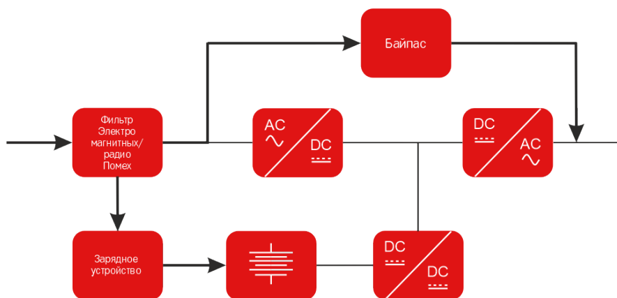
Рис. 3-3 Режим байпаса
